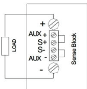
Local Sensing (fig.5)
